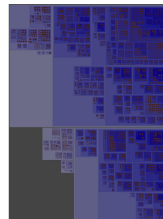
CodeCity
