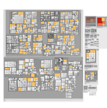
EvoCells Treemap
